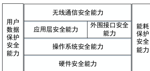
图 2 智能家居终端设备安全能力框架图
