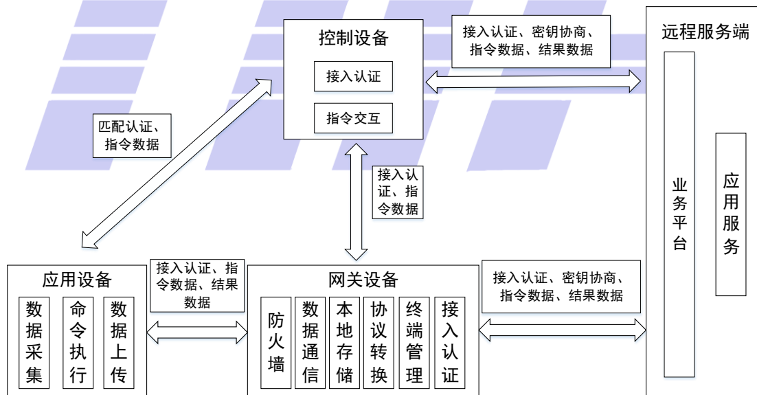
图 1 智能家居终端应用流程
