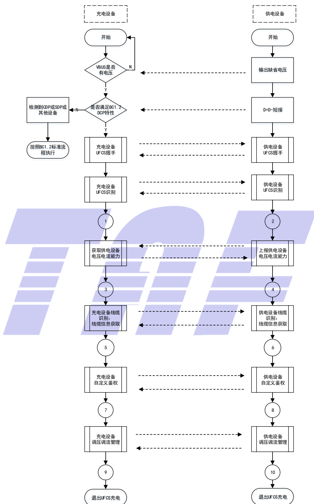
图 50 UFCS 工作流程总图
