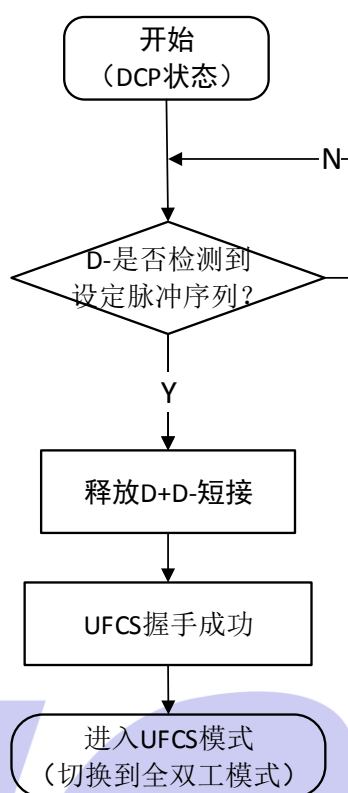
图 6 供电设备端 UFCS 握手检测流程
