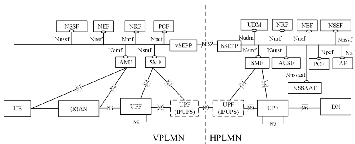
图 B. 4 基于服务接口的 5G 核心网漫游（归属路由方式）网络架构
