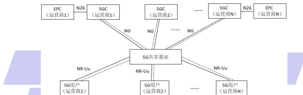
图 A.1 独立组网 (SA) 下 5G 接入网共享的网络结构 (各运营商 5GC 独立部署)
