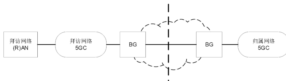
图 B.1 独立组网（SA）5G 核心网漫游的组网结构
