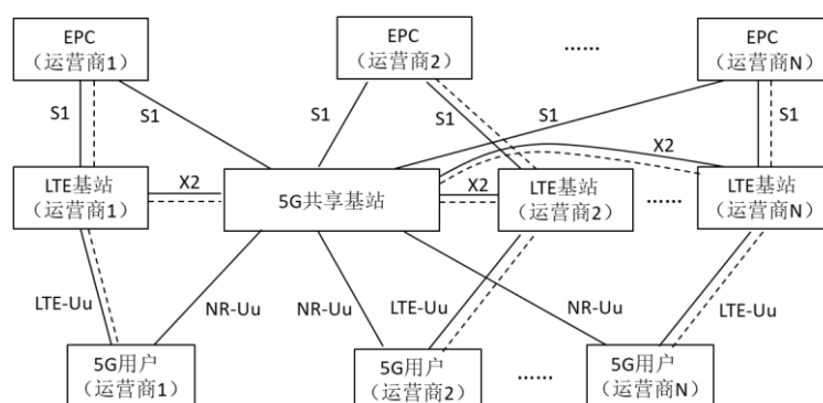
图 A.3 非独立组网 (NSA) 下 5G 接入网共享的网络结构 (情况 b)
