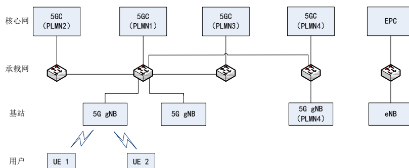
图 1 5G SA 接入网共享测试组网示意
