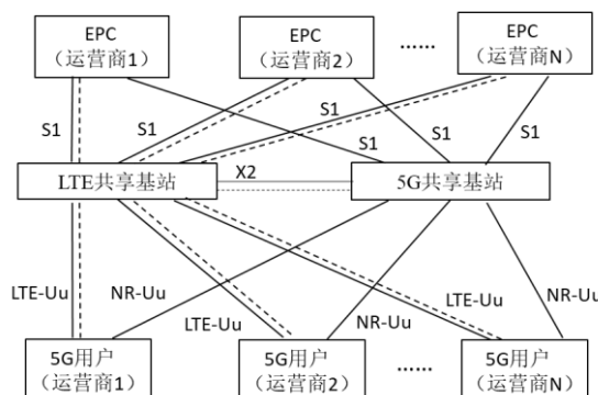
图 A.2 非独立组网 (NSA) 下 5G 接入网共享的网络结构 (情况 a)
