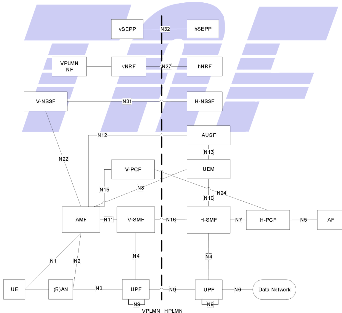
图 B.3 基于参考点的 5G 核心网漫游 (归属路由方式) 网络架构
