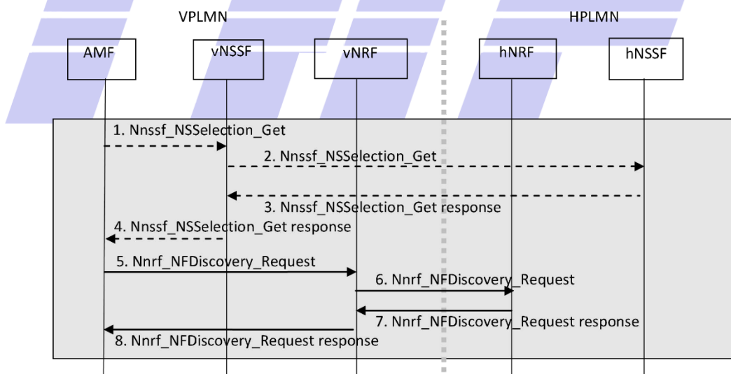
图 B.6 有 NSSF 参与的 hSMF 选择流程
