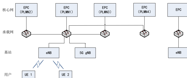
图 2 5G NSA 接入网共享测试组网示意
