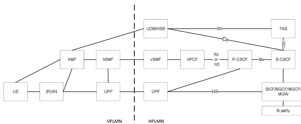
图 B.8 5G 核心网漫游 VoNR 业务网络架构
