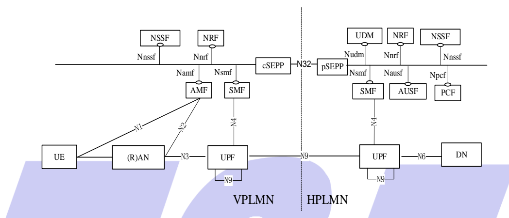
图 3 5G SA 核心网漫游组网架构图
