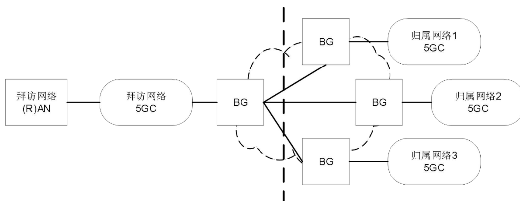
图 B.2 向不同运营商提供 5G 核心网漫游的组网结构
