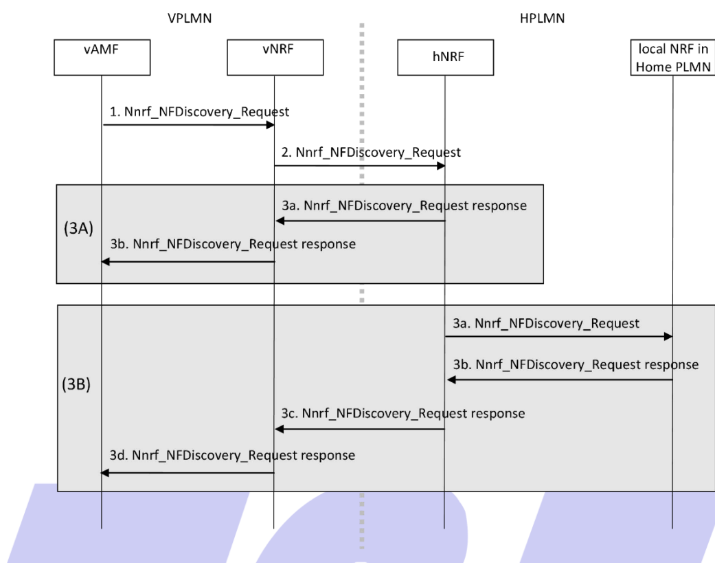
图 B.5 无 NSSF 参与的 hSMF 选择流程
