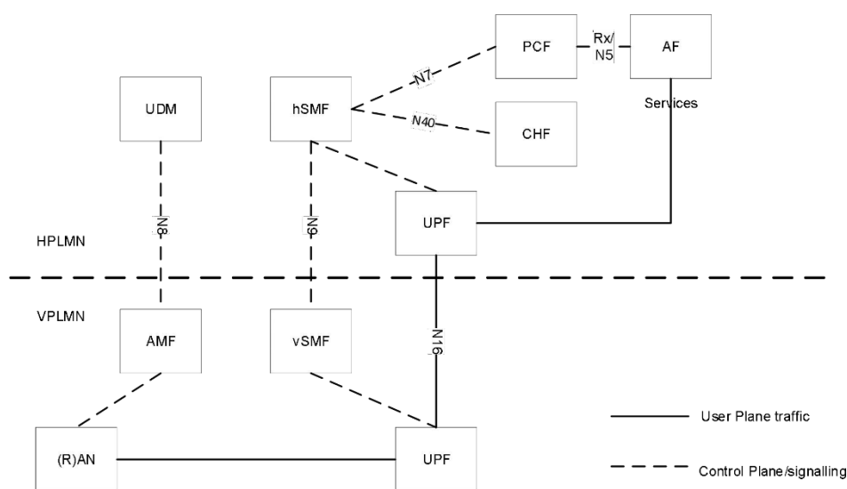
图 B.9 归属路由模式的服务质量控制模型
