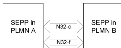
图 B.7 核心网漫游的 N32 接口
