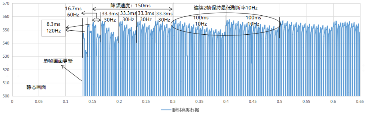
图10 降频速度亮度波形图示例
